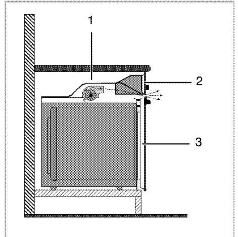
1 Soğutma fanı
